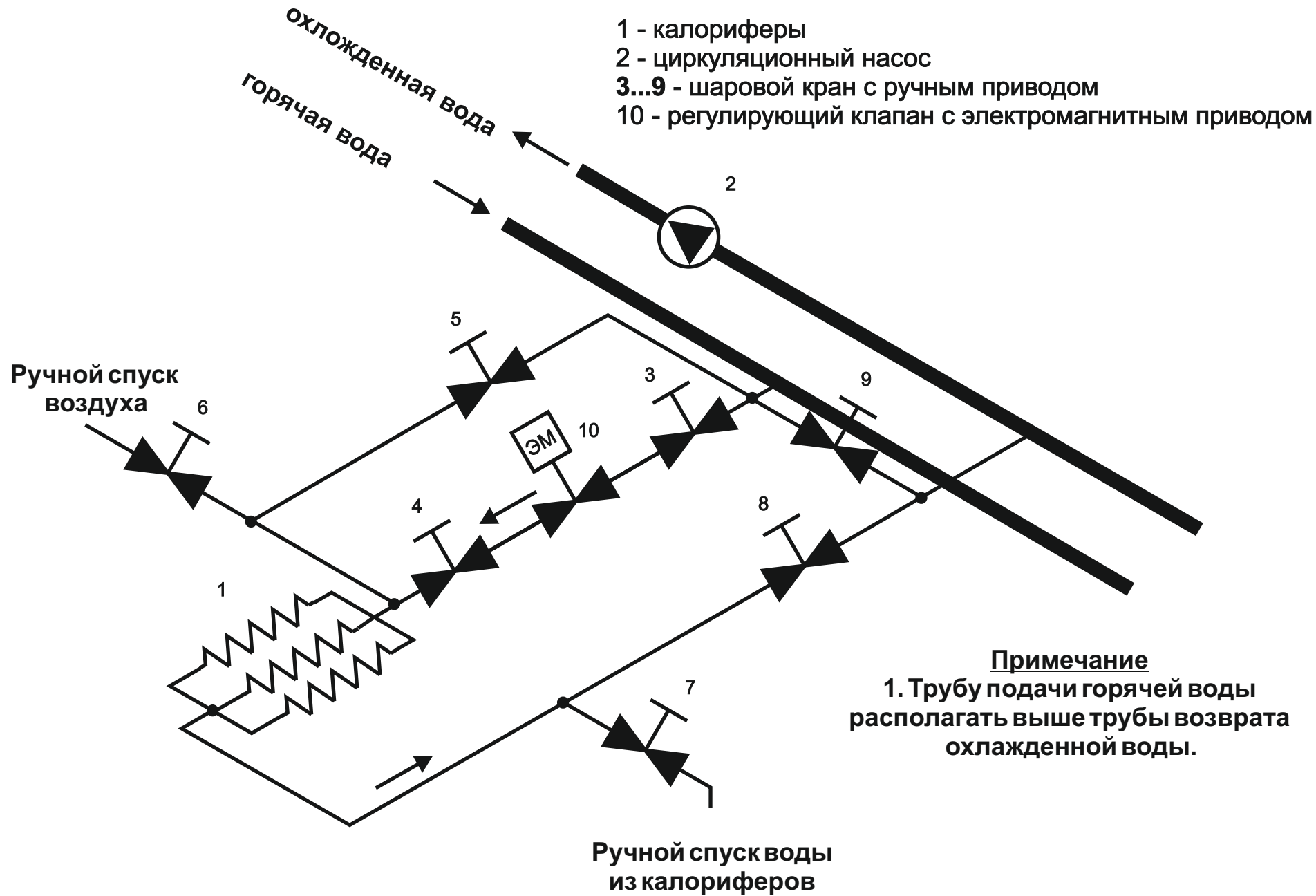
Схема снабжения горячей водой 1 сушильной камеры
